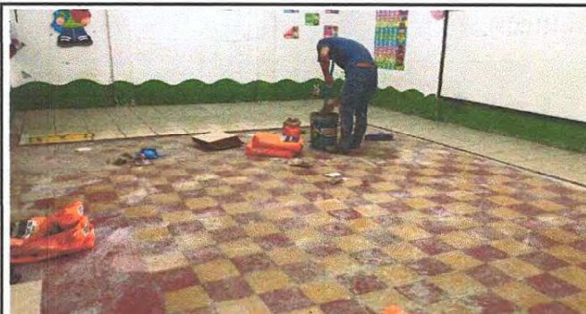
Foto 8: Piso, instalación de piso cerámico en el aula tres del primer nivel de la escuela.
