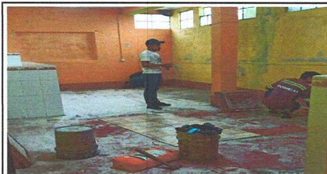
Foto 11: Piso, instalación de piso antideslizante en la cocina de la escuela.
